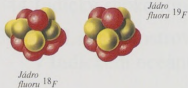
Izotopy
