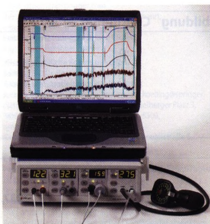
Messapparatur zur Messung der Mikroziirkulation durch Laser-Doppler-Fluxmetrie.
