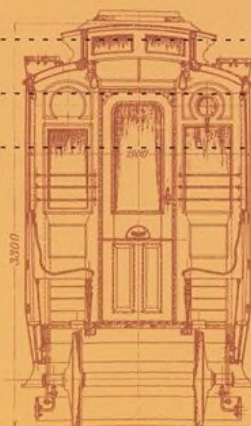
Trichwagen.
