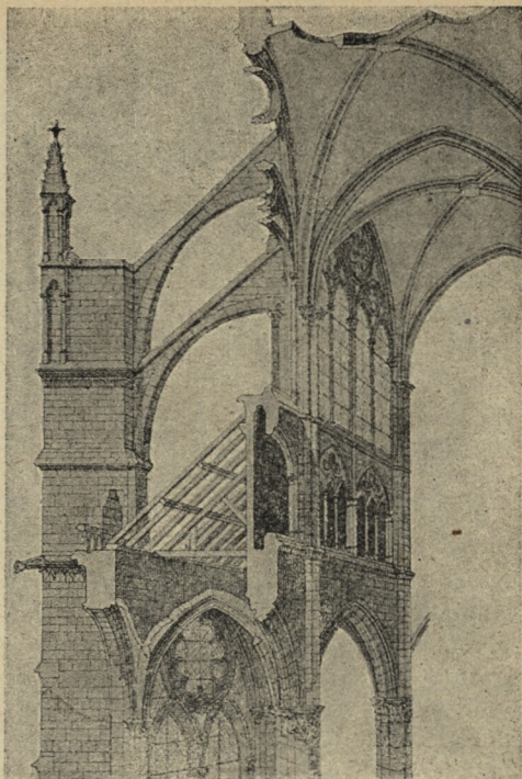
Obr. 16. Opěrný gotický systém. (Katedrála v Amiensu.)
