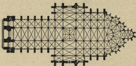
Obr. 17. Půdorys katedrály amienské. Chor je prodloužen. Boční lodi jsou spojeny ochozem, k němuž se druží věnec kaplí.
