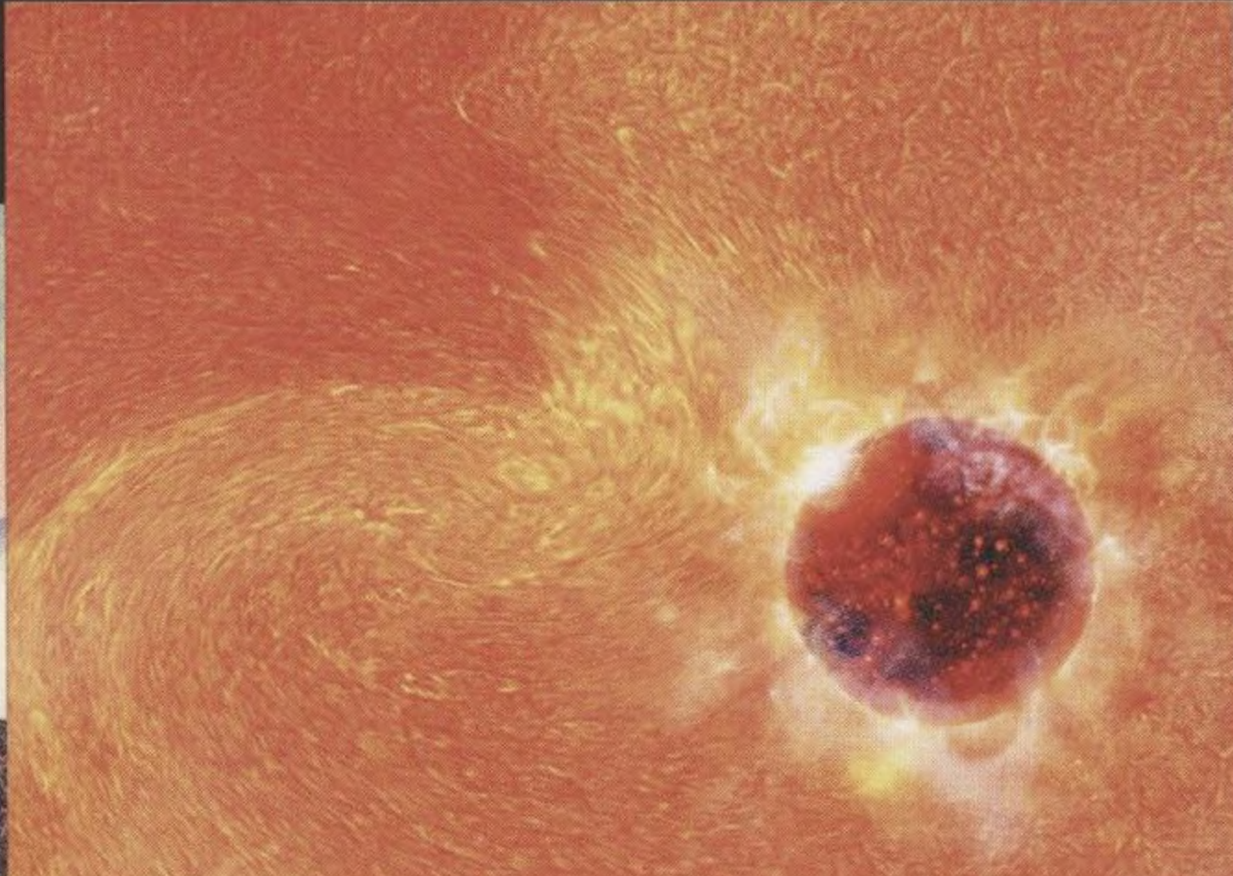
OD SOUČASNOSTI PO 13,8 MILIARDY LET PO VELKÉM TŘESKU
