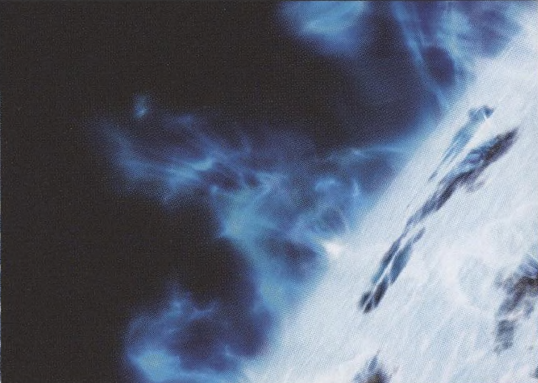
400 000 AŽ 700 MILIONŮ LET PO VELKÉM TŘESKU
