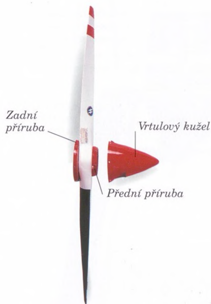
VRTULE MODERNÍHO LEHKÉHO LETADLA
