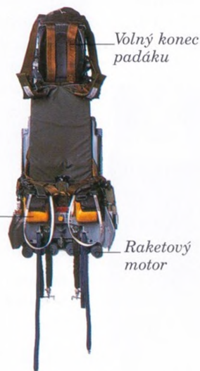
MODERNÍ VYSTŘELOVACÍ SEDADLO
