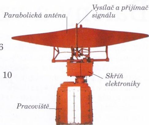
LETIŠTNÍ RADAR, 1953
